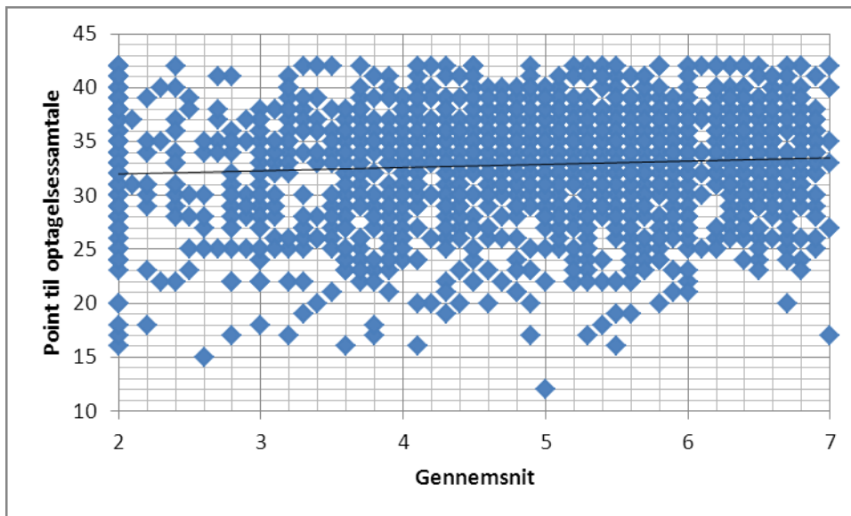
Diagram 5: Regression af karaktergennemsnit og point.
