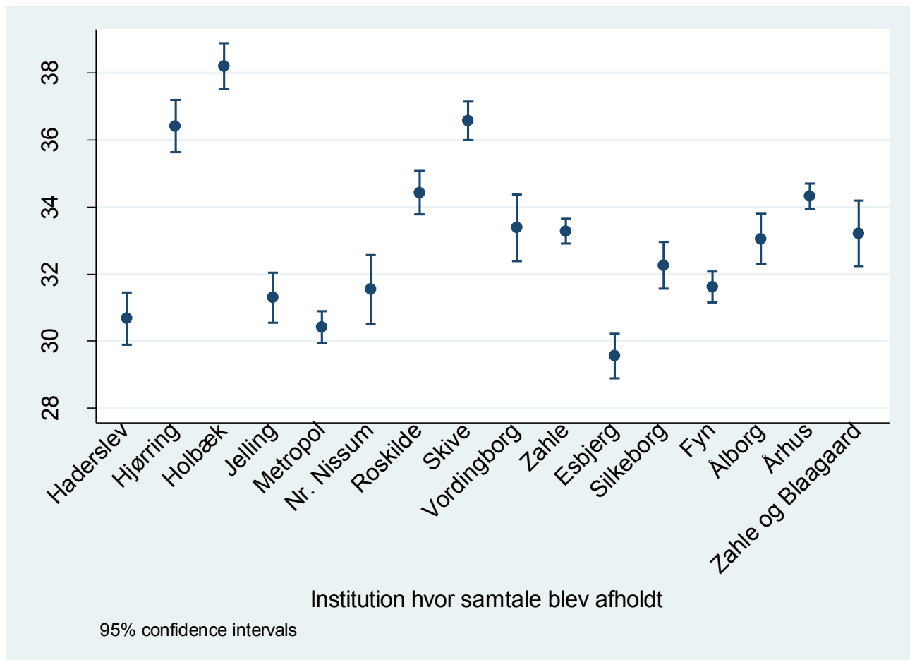
Diagram 1 – konfidensintervaller for de enkelte prøvesteder:
