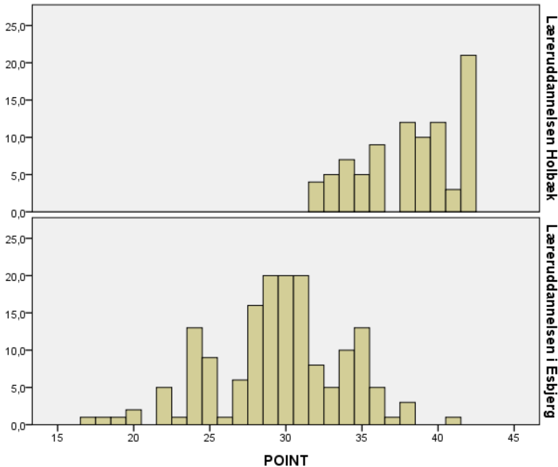
Diagram 3-4 – Pointfordeling på Holbæk og Esbjerg
